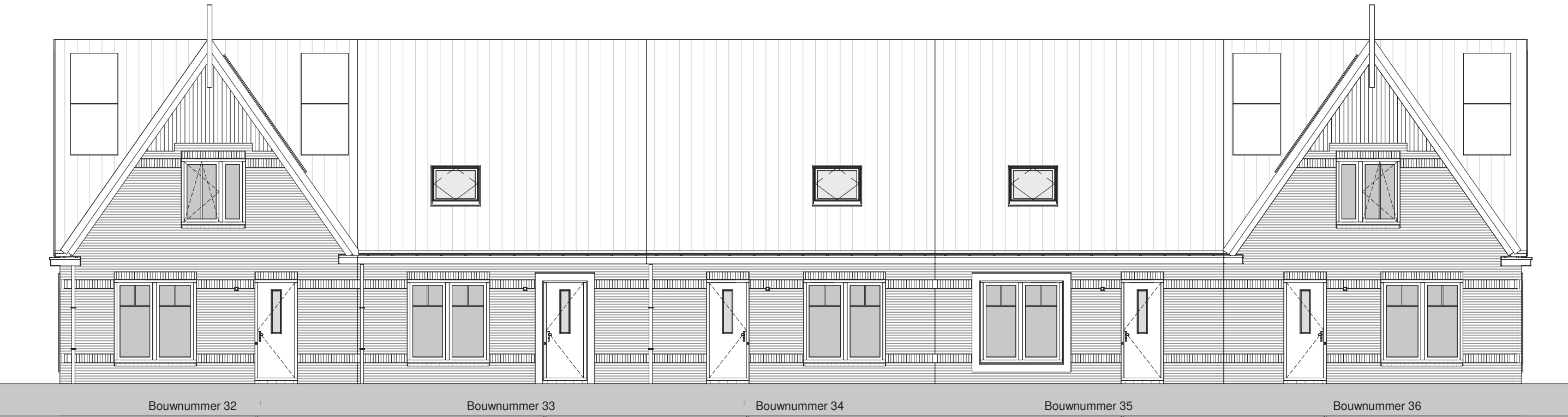
voorgevel 1:100
